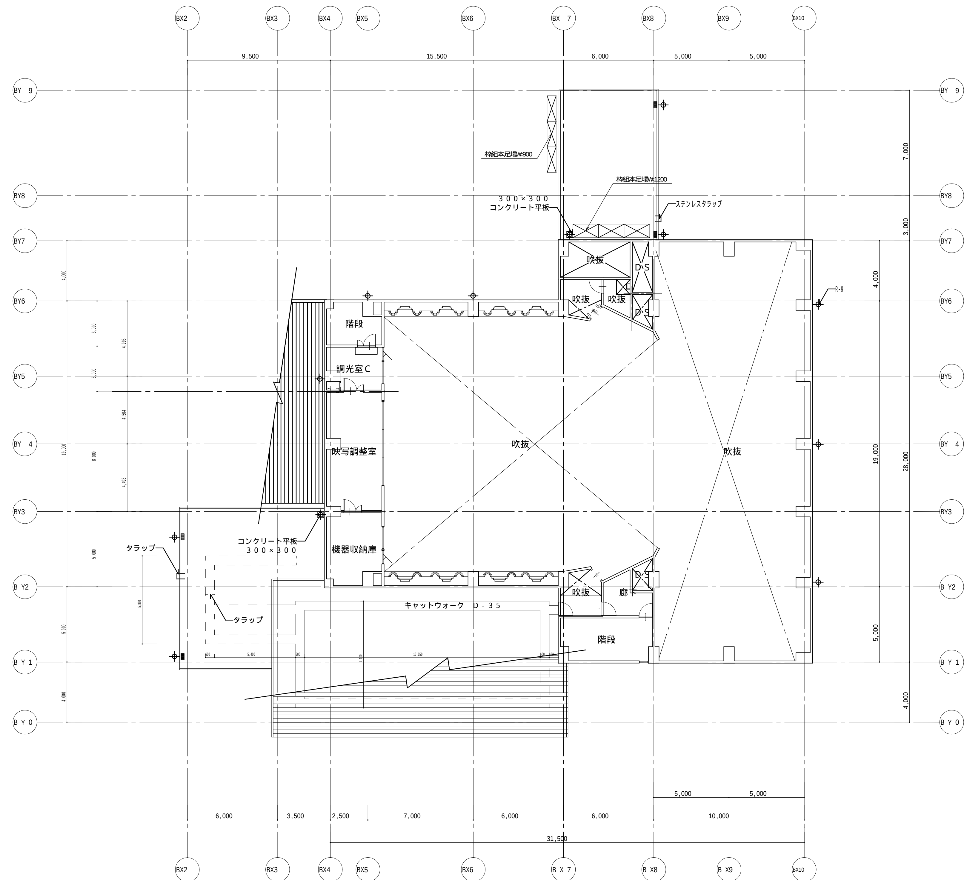
Z7 2階上部平面図 S:1/150
