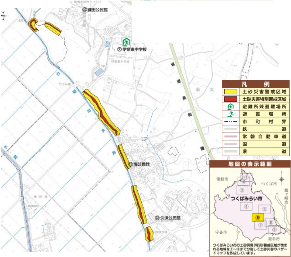
図：土砂災害警戒区域及び土砂災害特別警戒区域（板橋・南太田地区）
