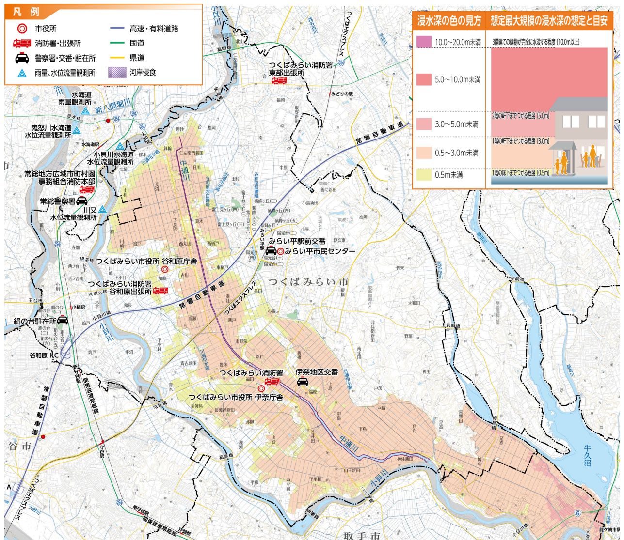
図：中通川氾濫推定区域図
