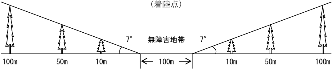
図：発着場における無障害地帯 (着陸点)
