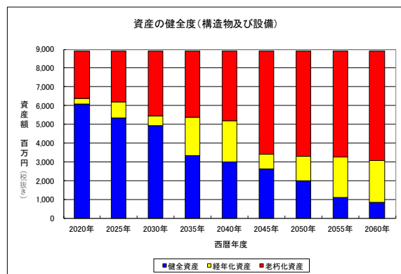
図 4. 2. 1 資産の健全度 (構造物及び設備)
