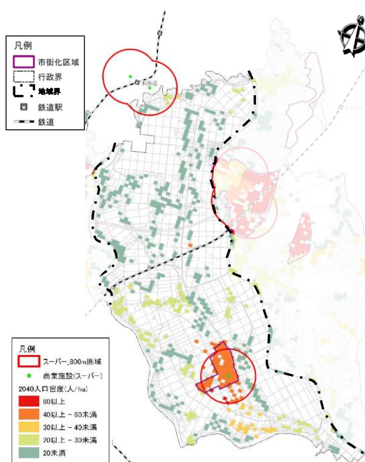
■ 商業施設の徒歩圏人口カバー圏(2040 年度)
