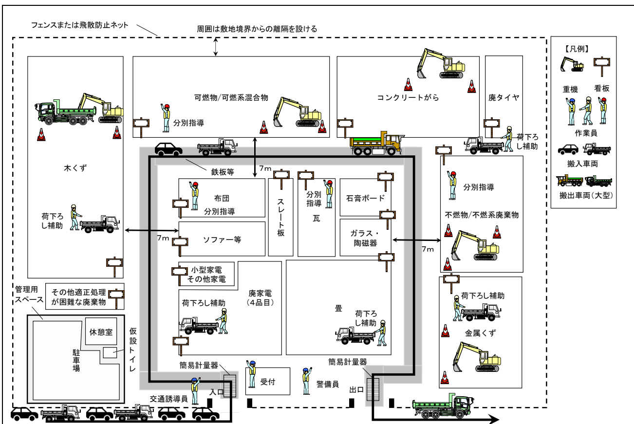
図表39 一次仮置場の配置計画（レイアウト）例
