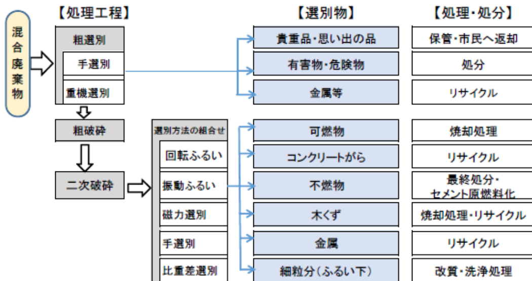
図表43 混合廃棄物の処理（例）
