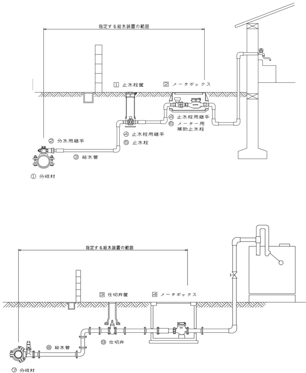
図一8.1 指定する給水装置の範囲
