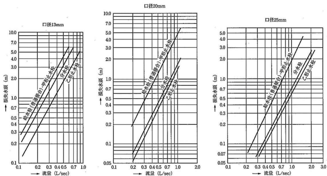
図-6.5 止水栓類の損失水頭
